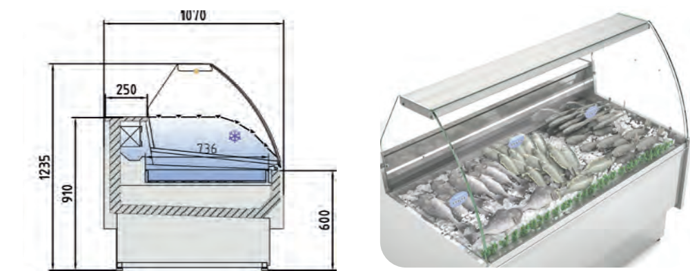
Detalle plano de exposición cuba hermética Detail of the airtight container display plan
