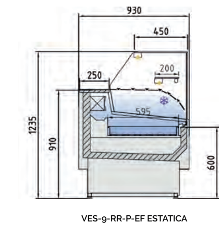
Detalle plano de exposición cuba hermética Detail of the airtight container display plan
