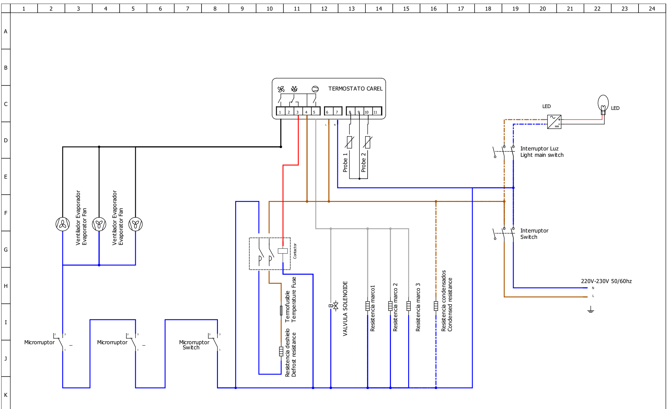
ESQUEMA ELECTRICO DRVC-2003 PREINSTALACION
